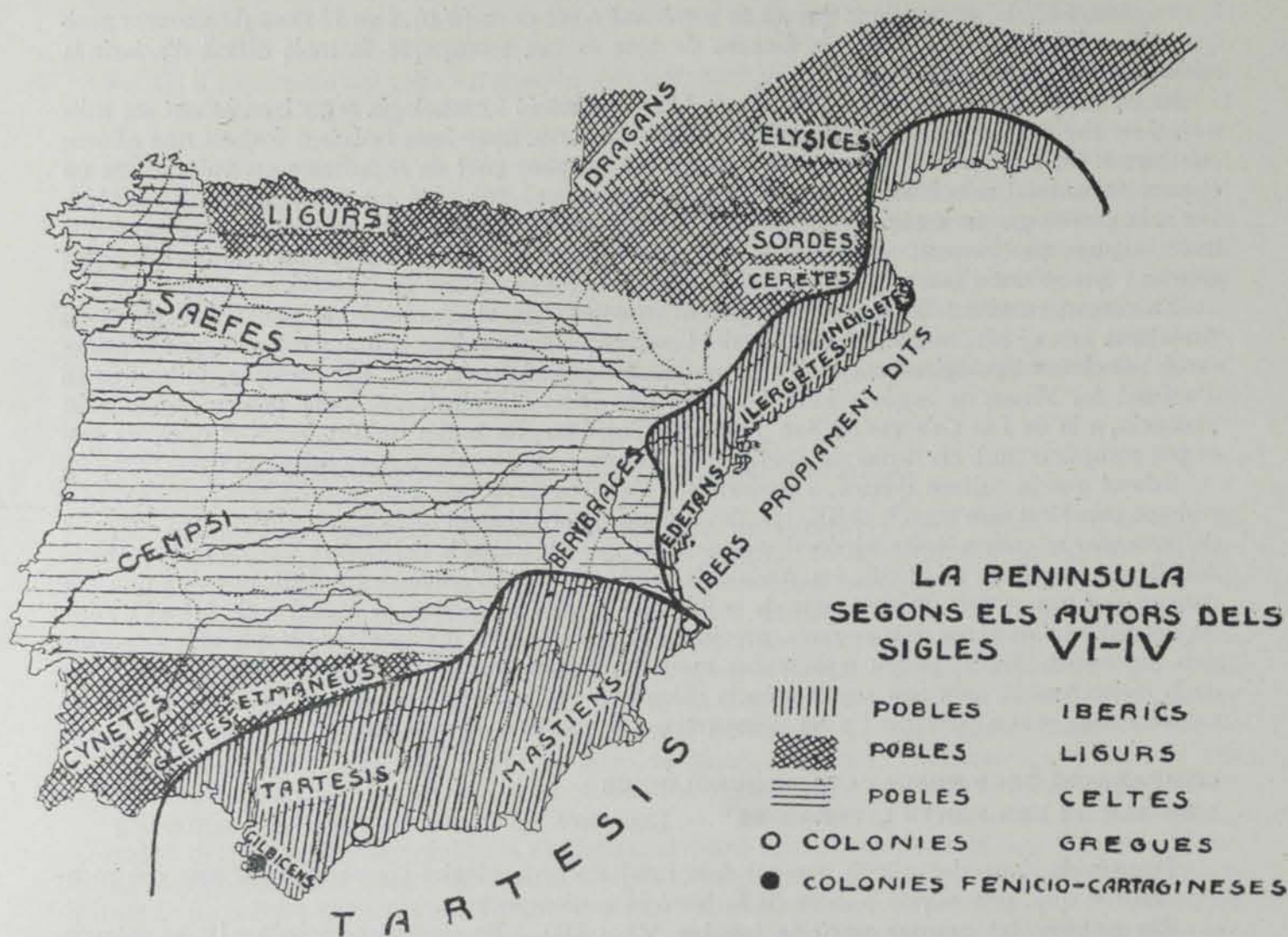
Fig. 521. — La etnologia de la península segons les fonts literàries (primer període)
