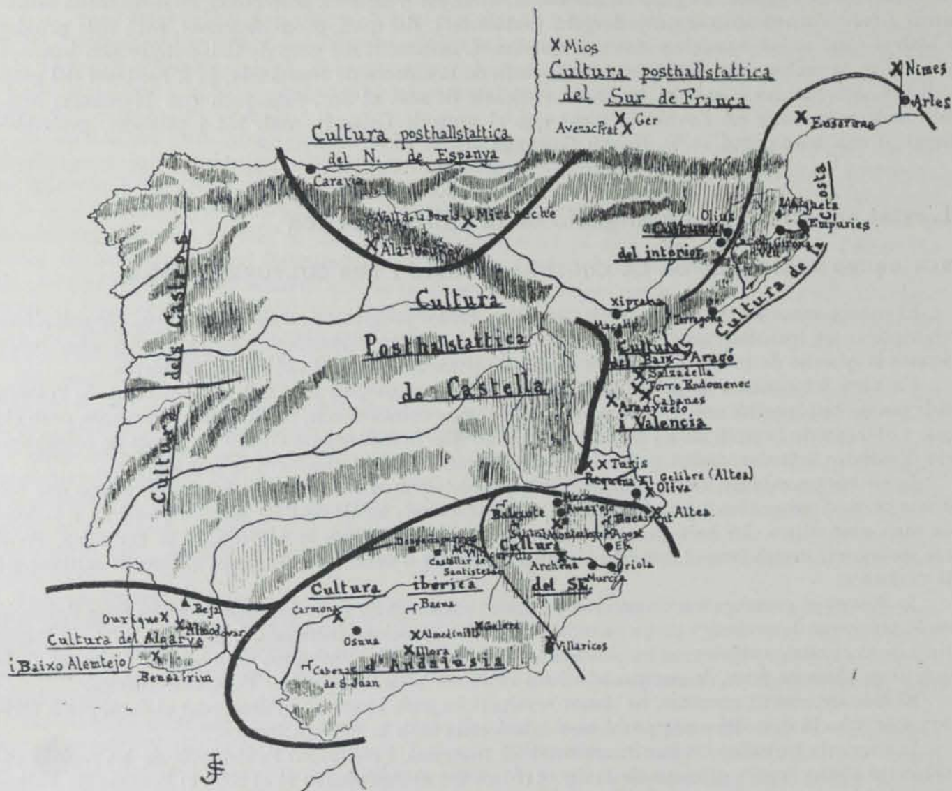
Fig. 516. — Els grups de la cultura ibèrica i les civilitzacions veïnes del segle V al III
